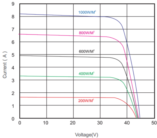
Зависимость электрических параметров от интенсивности солнечного света
